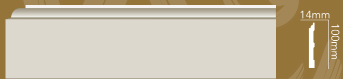
WA-PF084 L:2400mm W:100mm
