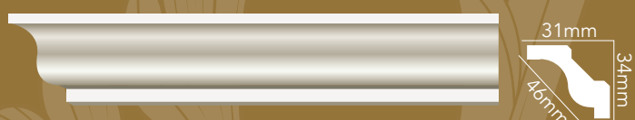
WA-PC064 L:2400mm W:46mm
